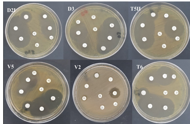
Figura 3. Identificación de mecanismos de resistencia de B. gladiolii y B. plantarii . D: aislados finca La Doña; T: aislado centro experimental TAINIC; V: aislados finca Virginia; 2, 3, 5 y 6: número de aislado; I y II: número de placas.
