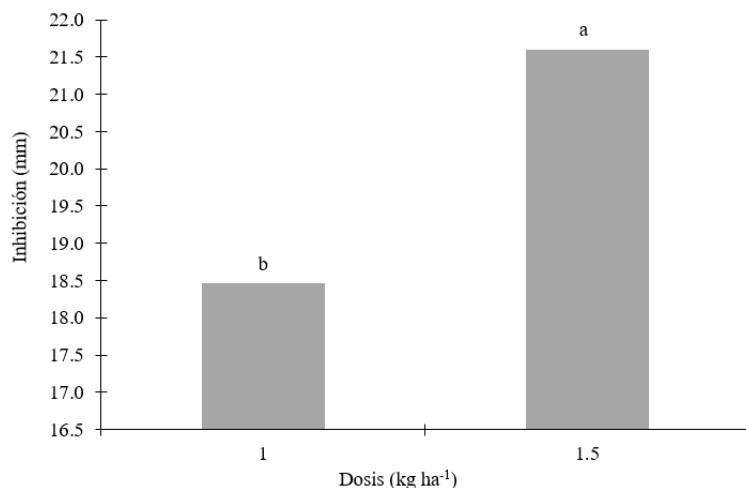
Figura 6. Sensibilidad de B. gladiolii y B. plantarii según dosis de ácido oxolínico.
