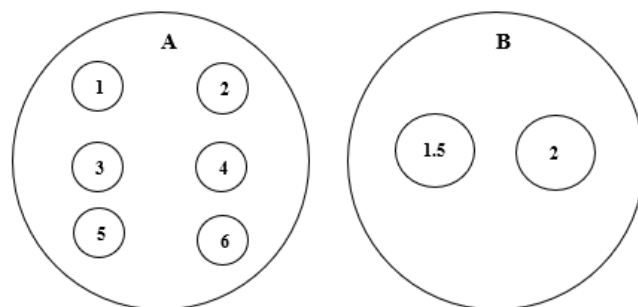
Figura 2. Posición de los bactericidas comerciales para prueba de sensibilidad.
