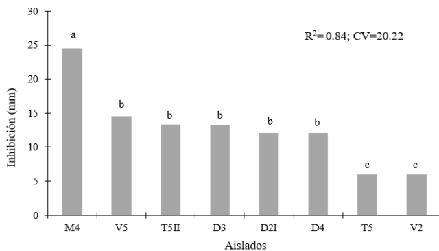
Figura 7. Sensibilidad de B. gladiolii y B. plantarii al ácido oxolinico más gentamicina.
