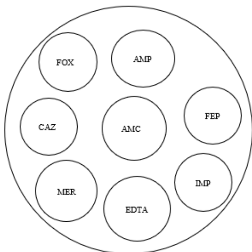
Figura 1. Orden de los antibióticos para la identificación fenotípica de mecanismos de resistencia de B. gladiolii y B. plantarii .
