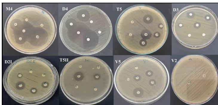
Figura 4. Aislados de Burkholderia gladiolii y Burkholderia plantarii en medios de cultivo Mueller-Hinton.
