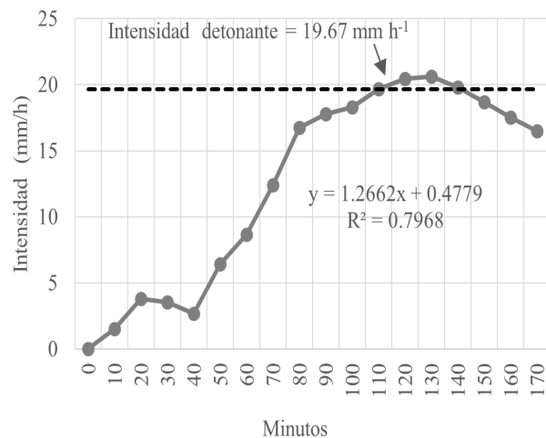
Figura 12. Curva de masa de intensidad del evento lluvioso del 3.oct.16.
